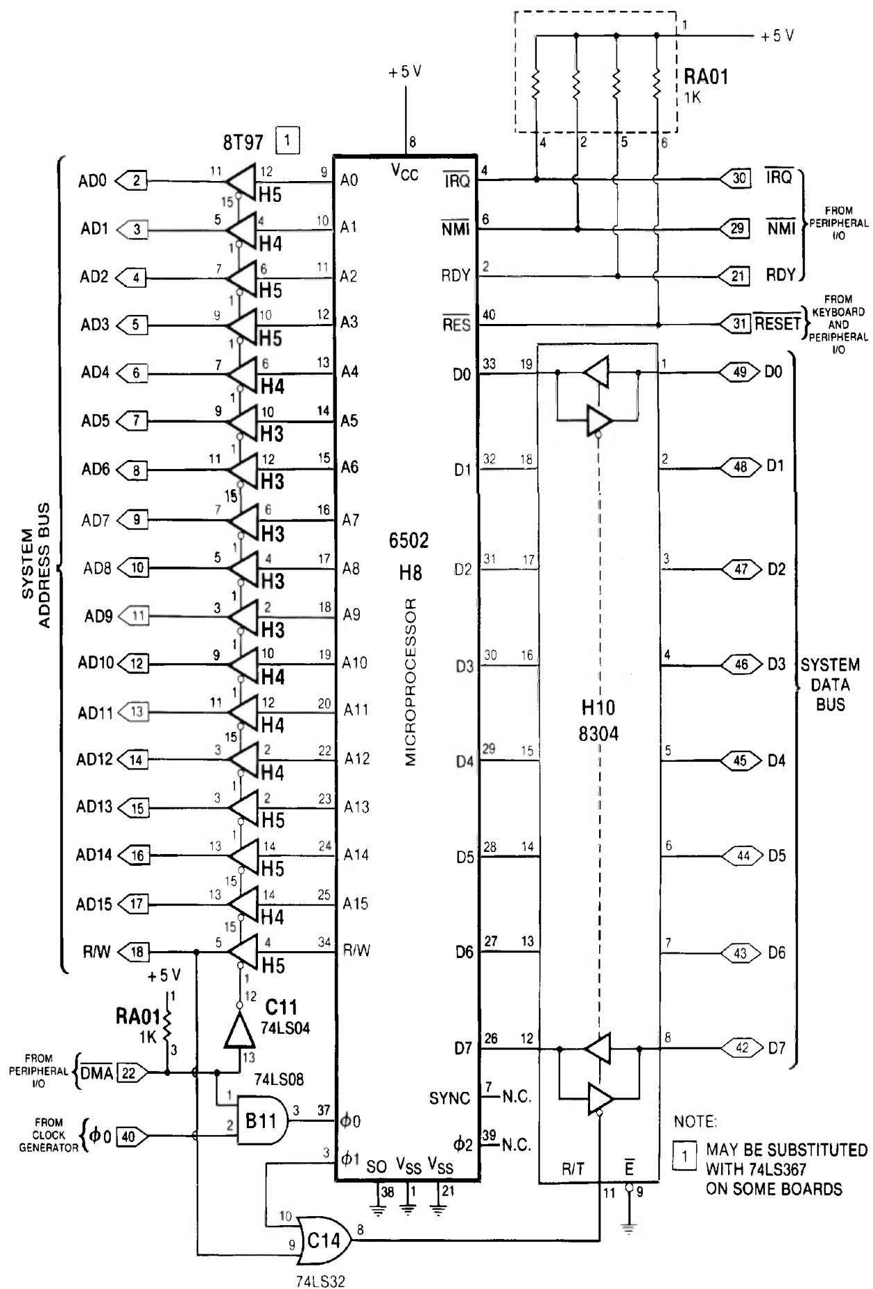
Fig. C-8. Microprocessor (RPI).
