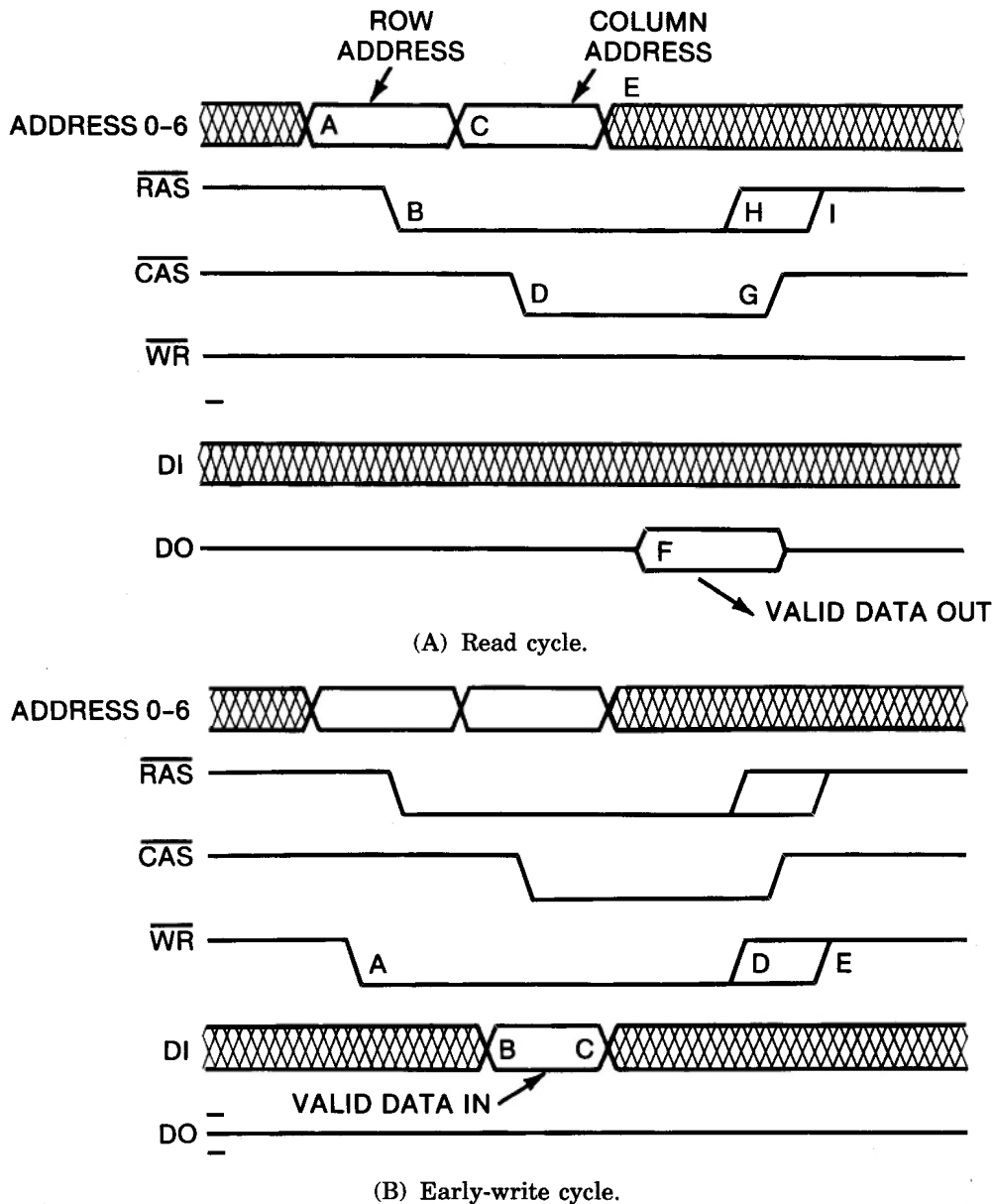
Fig. 5-1. 4116 RAM cycles.
