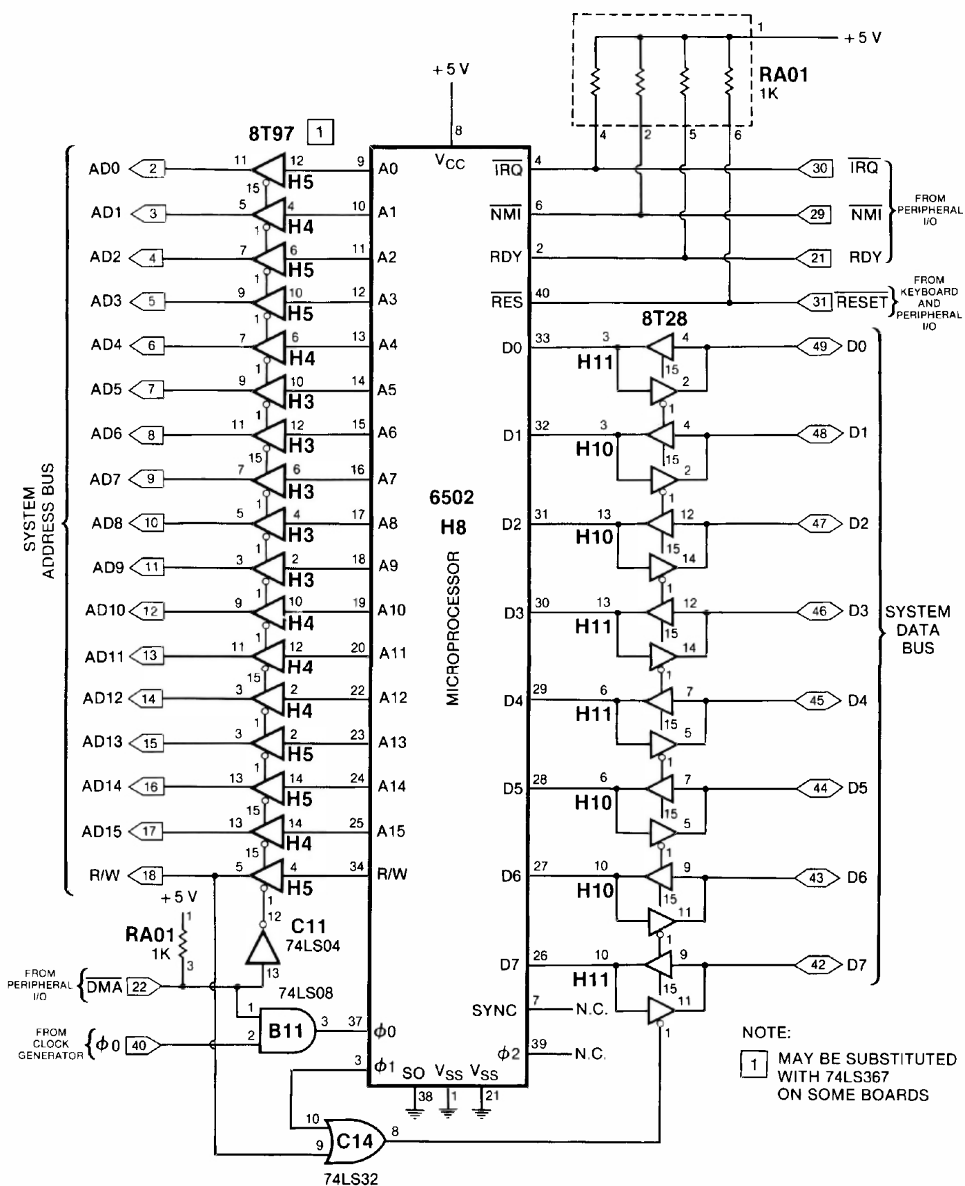
Fig. C-8. Microprocessor (Rev. 0,1,7).
